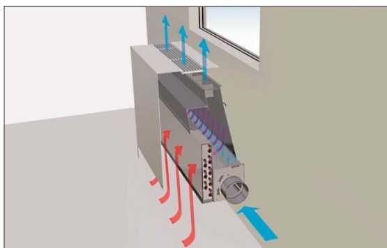
Schema Induktionsgerät
