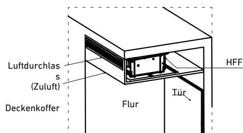
Isometrische Ansicht
