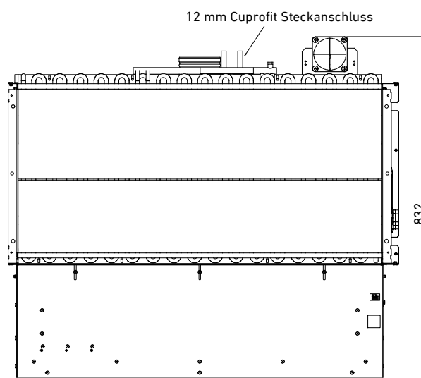
Untersicht
