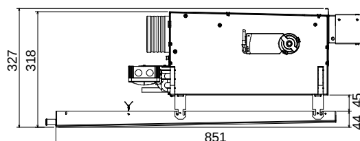
Seitenansicht von links
