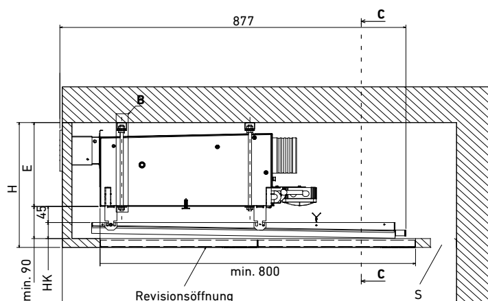
Seitenansicht rechts
