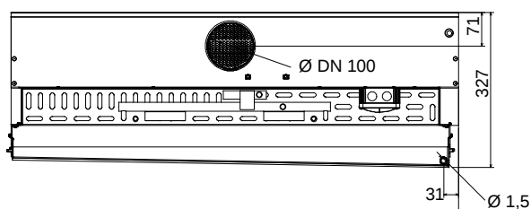
Rückansicht
