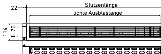
Vorderansicht
