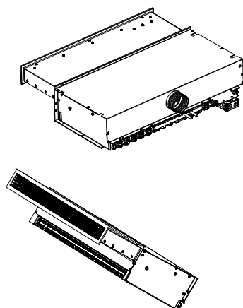
Isometrische Ansichten
