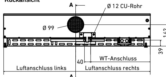
Rückansicht
