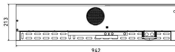
Rückansicht
