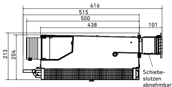
Schnitt A-A
