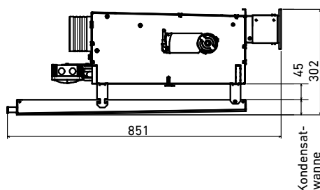
Vorderansicht
