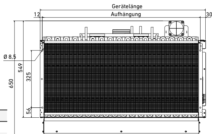
Untersicht
