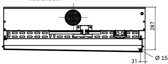
Rückansicht
