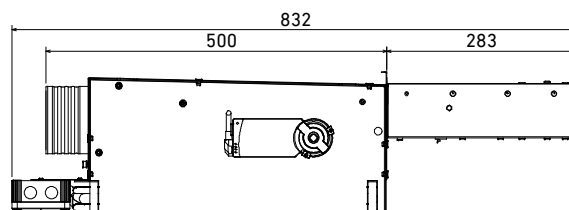
Seitenansicht von links
