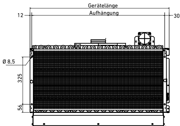
Untersicht
