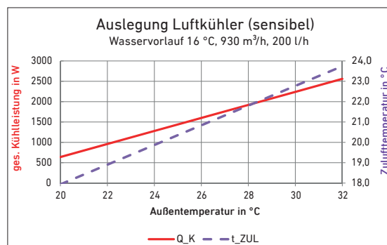
Abbildung 26a: Auslegung Luftkühler
