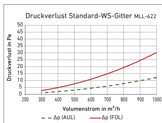
Abb. 21: Auslegung Wetterschutzgitter mit 50mm-Teilung
