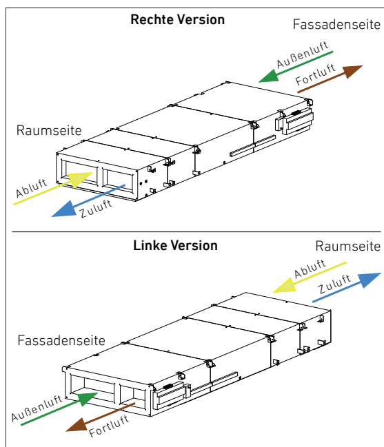
Abb. 16: Definition für rechtes und linkes FVS-1000/DI-Gerät
