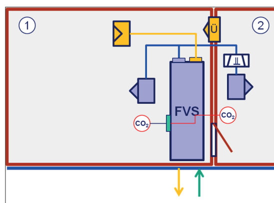
Abb. 27: Ein FVS-1000-Gerät versorgt einen Haupt- und einen Nebenraum
