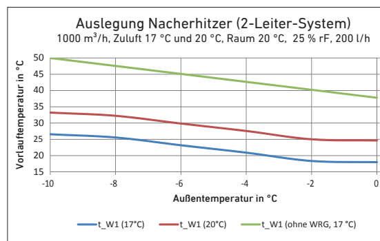
Abbildung 25b: Auslegung Nacherhitzer
