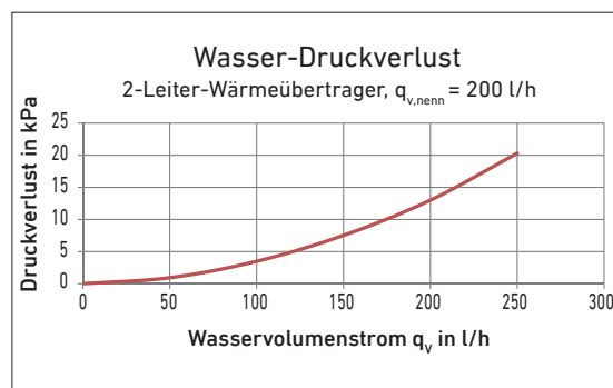
Abbildung 26b: Wasserseitige Druckverluste (2-Leiter-System)
