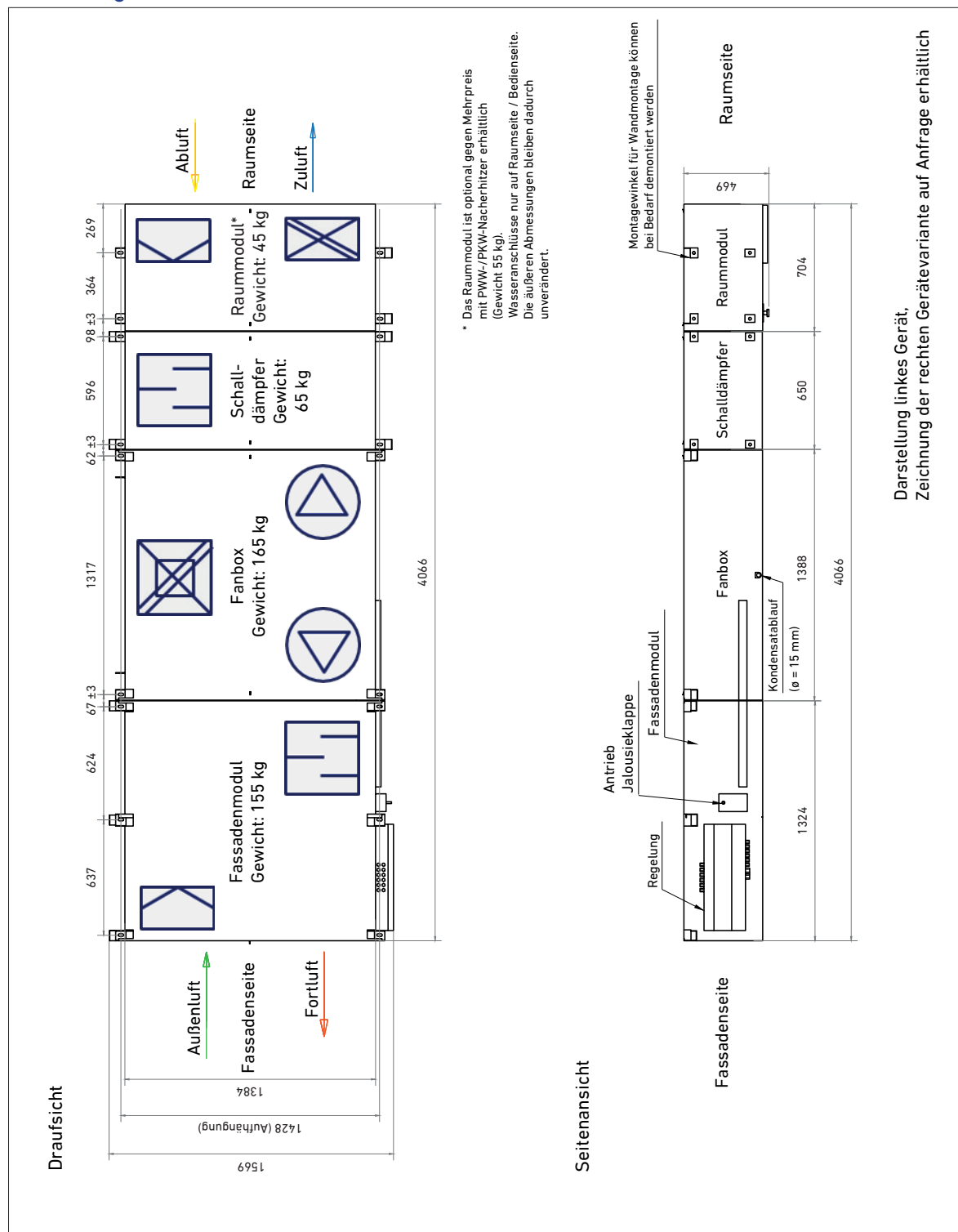
Abb. 10: Abmessungen FVS-1000/DI (linkes Gerät)
