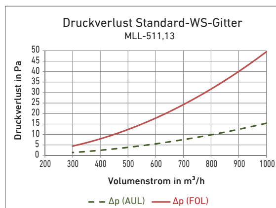
Abb. 20: Auslegung Wetterschutzgitter mit 33mm-Teilung
