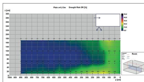
Abb. 8: Zugluftbewertung bei 930 m 3 /h und 7 K Zuluftuntertemperatur (max. Kühlfall) Zugluftbewertung
