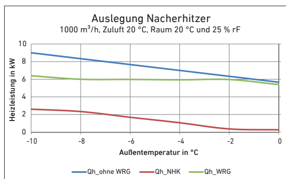
Abbildung 25a: Auslegung Nacherhitzer
