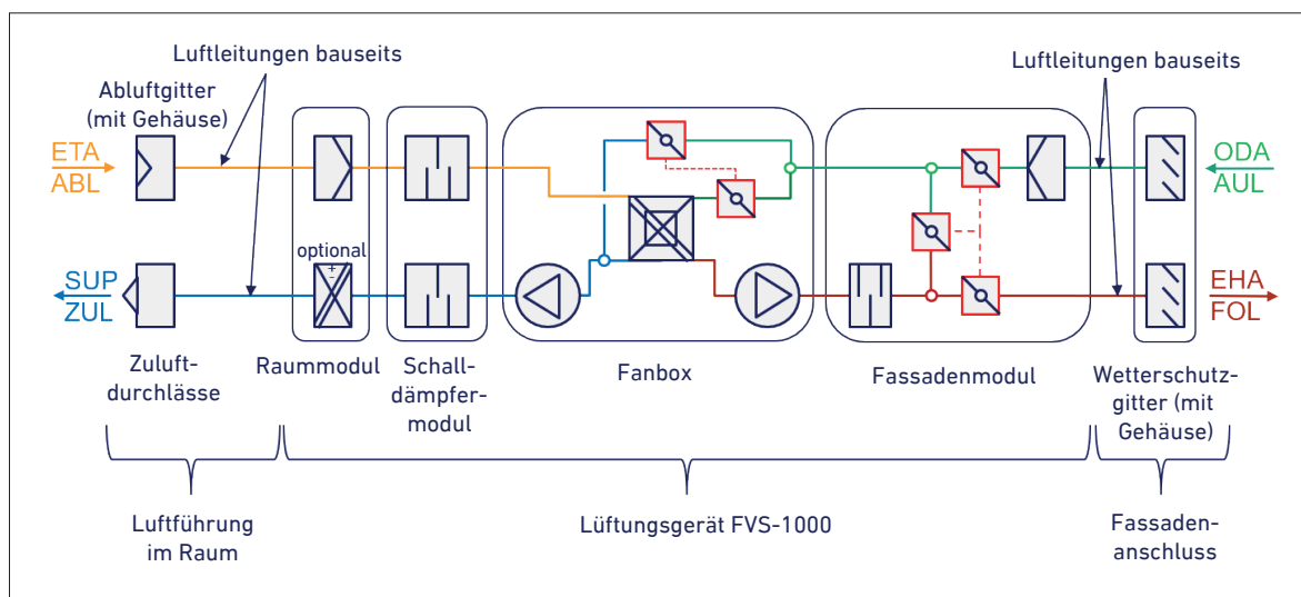
Abb. 2: Lüftungsschema
