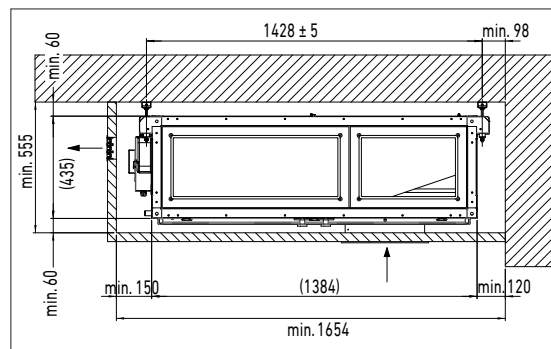
Abb. 12: Schnitt durch Deckenkoffer mit Zuluftplenum. Ansicht Fassadenseite.
