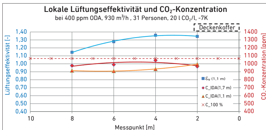
Abb. 9: CO 2 -Konzentration und lokale Lüftungseffektivität
