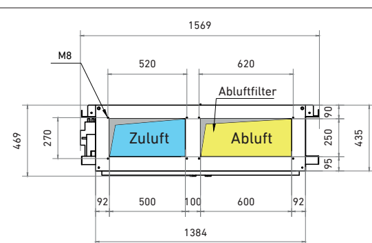
Linkes & rechtes Gerät: Zuluft Raum-/Bedienseite, Abluft Wandseite
