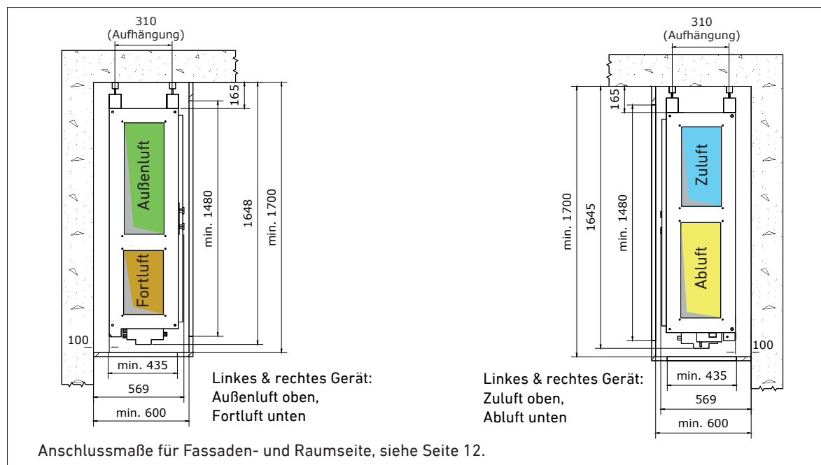
Abb. 13a: Abmessungen und Anschlüsse Luftleitungen (linkes Gerät)
