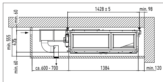
Abb. 11: Schnitt durch Deckenkoffer mit angeschlossenem Zuluftdurchlässen
