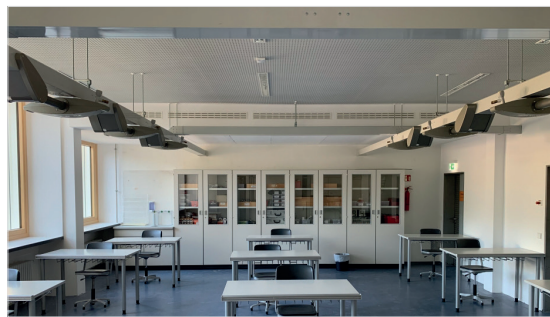
Einbau im Deckenkoffer. Dieser Einbau ist nur durch die hoch-induktiven Schlitzdurchlässe zugfrei realisierbar.
