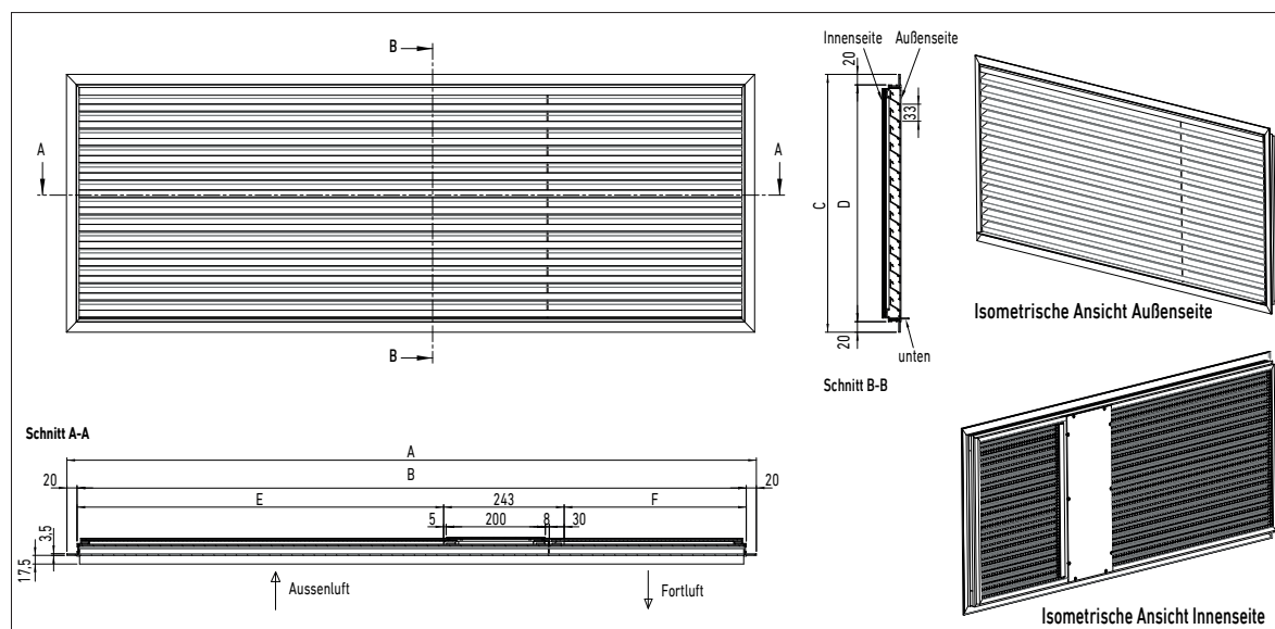
Abb. 19: Maßbild Wetterschutzgitter mit 33mm-Teilung (Typ FVS-1000/DI)
