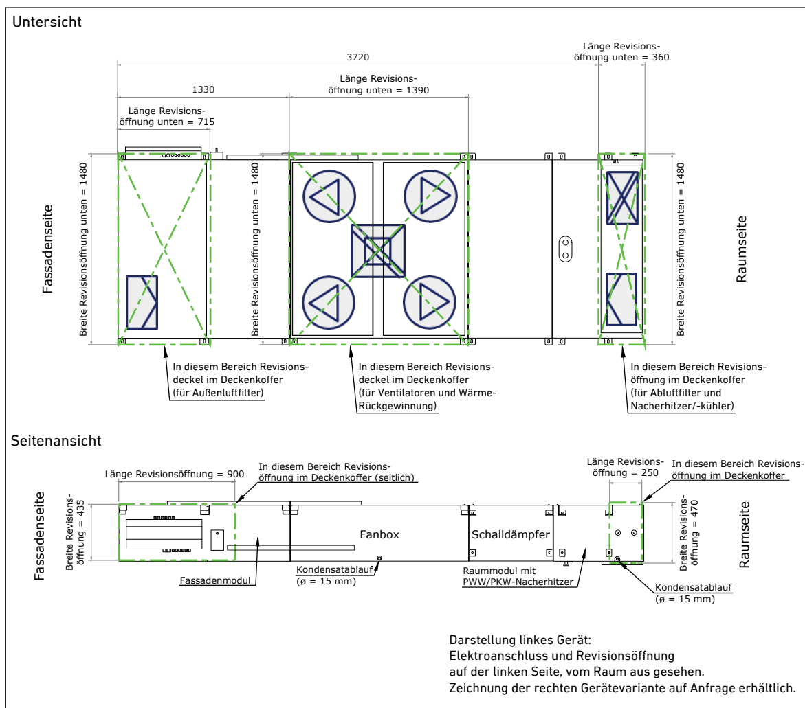
Abb. 14 Vermaßung der Revisionsöffnungen (grün umrandet, als Mindestgrößen vermaßt)
