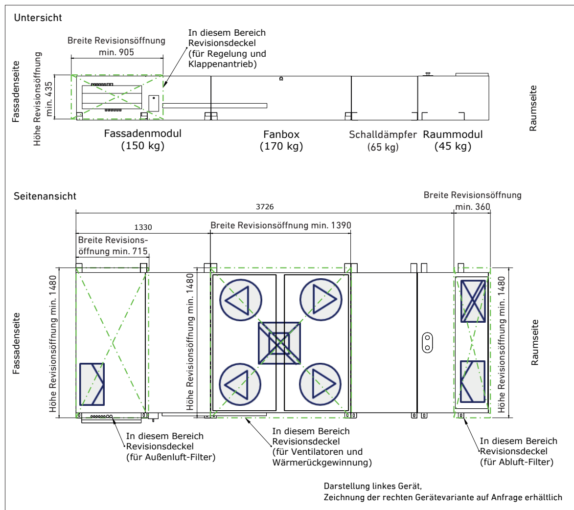
Abb. 15: Vermaßung der Revisionsöffnungen (grün umrandet, als Mindestgrößen vermaßt)
