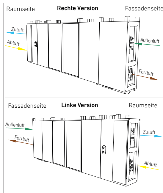
Abb. 17: Definition für rechtes und linkes FVS-1000/W-Gerät
