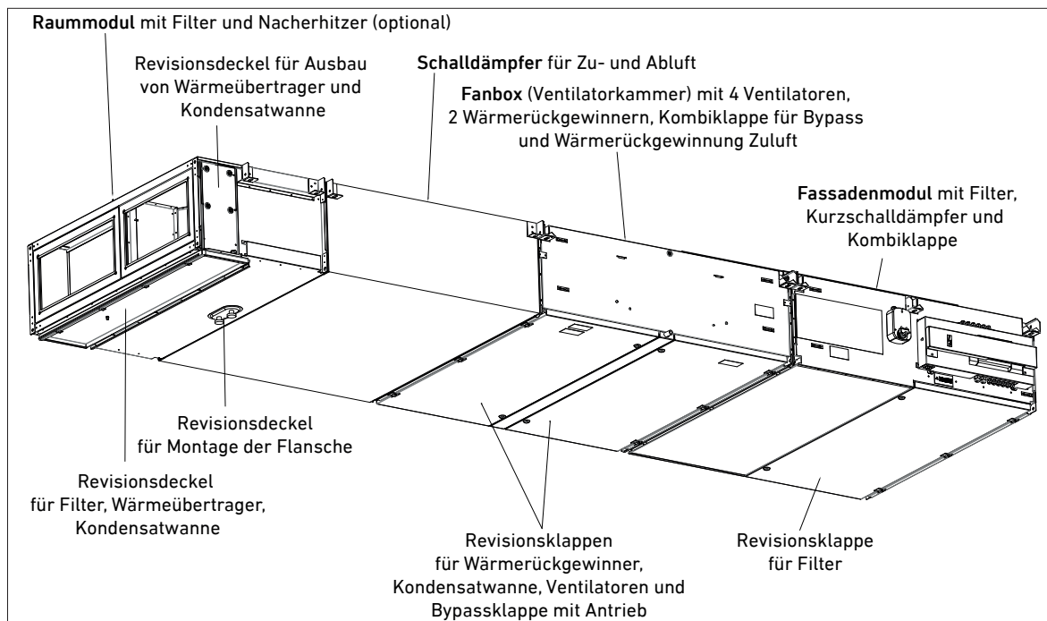
Abb. 1: Geräteaufbau ohne Anschlüsse auf Raum- und Fassadenseite
